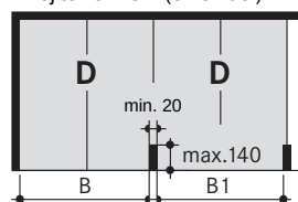
Dvojitě zařízení (6 vozidel)
